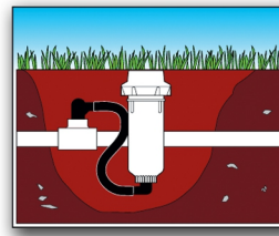
PVC 管及三通的安装位置不会影响到喷头最后的安装效果
